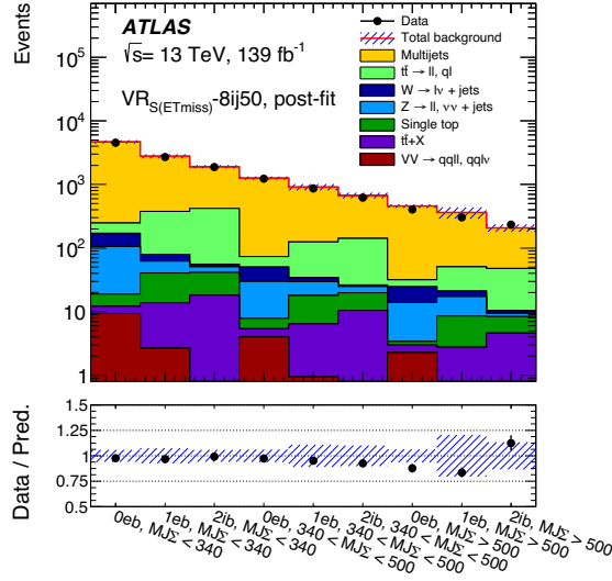
(b) VR_{S(E_{T}^{miss})}
