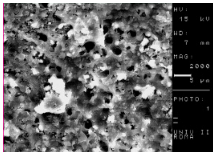
Fig. 5 - EDTA al 17% terzo apicale 5' 2000x.
