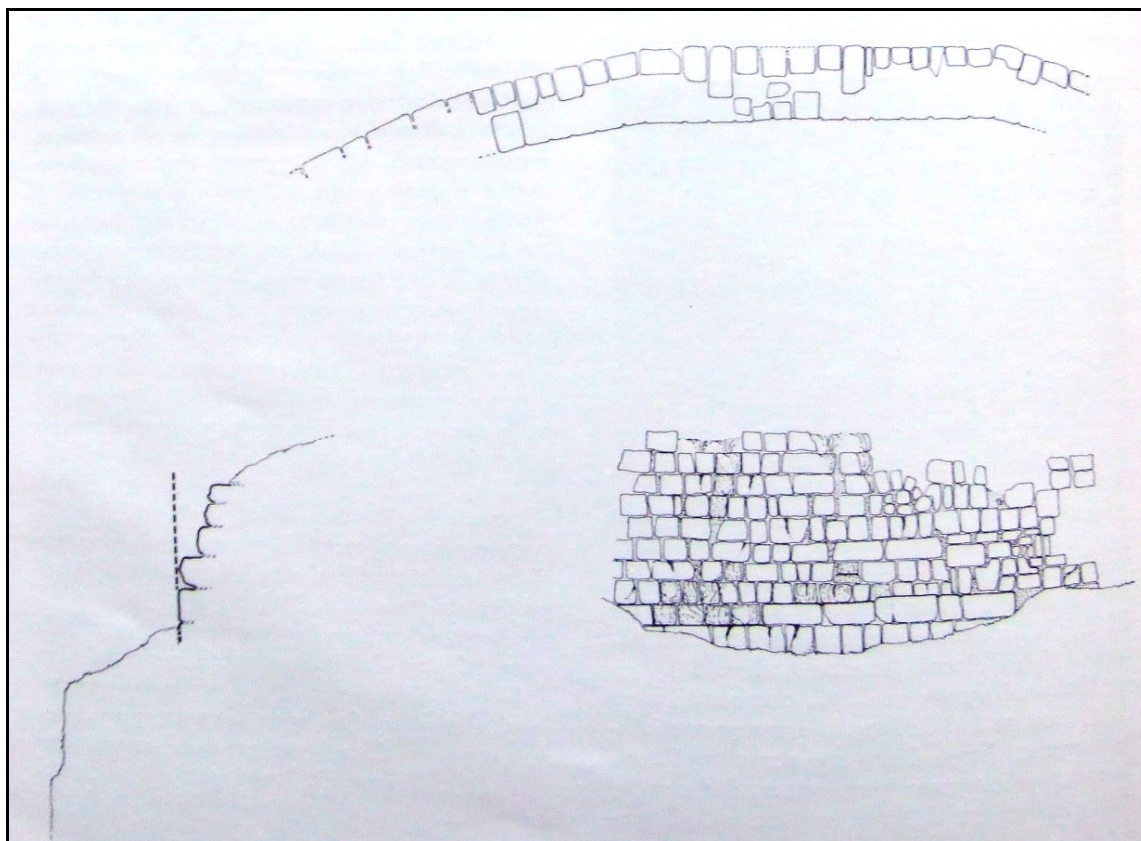
Fig. 43 – Mura urbane, Tratto 3: pianta e prospetto (da Morselli-Tortorici 1982)
